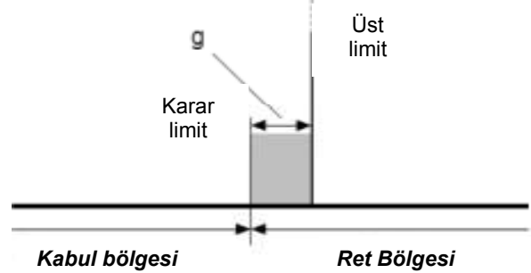
Şekil 2. Üst limit özelliklerine dayanan kabul ve ret bölgesi, karar limiti ve koruma bandı ( g ), ve doğru kabulün yüksek güvenilirliğine dayalı bir karar kuralı
