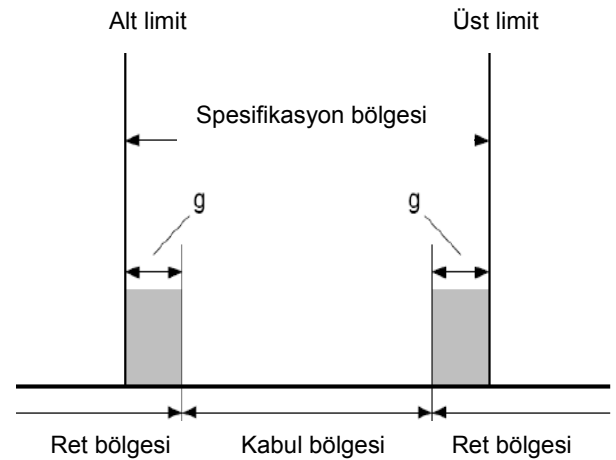
Şekil 4. Spesifikasyonda belirtilen üst ve alt limitler ve yüksek güvenilirlik ile kabul kararı alınmasını sağlayan bir karar kuralı ile belirlenmiş koruma bantları (g), karar limitleri, bir kabul bölgesi ve iki ret bölgesi
